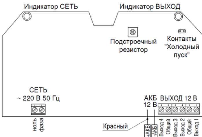
Рисунок 2 - общий вид платы изделия
